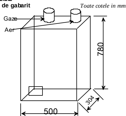
Fig. 2.1.2 Cote de gabarit
